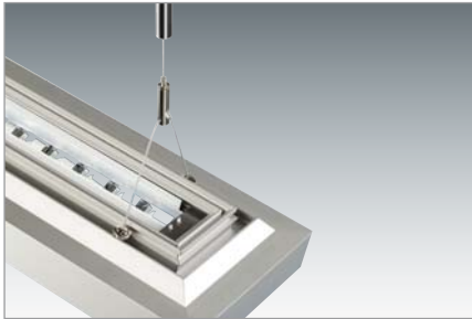
Dreipunkt-Seilaufhängung. 2 Stück für 1-längige Leuchte, mindestens 2 Stück für 2-längige Leuchte, mindestens 3 Stück für 3-längige Leuchte.
