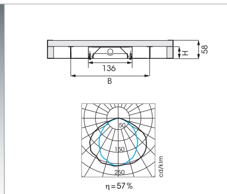
Luminaire encastré, rayonnement direct avec grille à lamelles.
