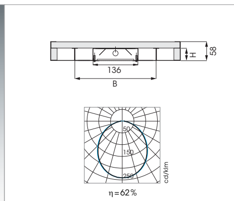
Luminaire encastré, rayonnement direct avec plaque diffuseur opale.
