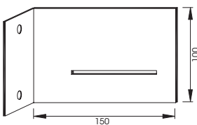
75-dur 010-00 dur-Wandtraverse
