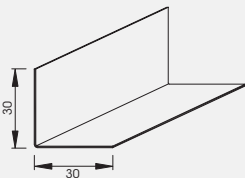
75-dur 009-00 dur-Wandanschlusswinkel
