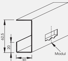
75-durprof-10 dur-Randtrageprofil R1
