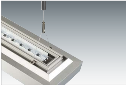
Dreipunkt-Seilauflhängung. 2 Stück für 1-längige Leuchte, mindestens 2 Stück für 2-längige Leuchte, mindestens 3 Stück für 3-längige Leuchte.
