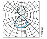
2xT5 \eta=76\%
