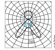
1xT5 \eta=65\%
