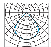
2 x T5 η=54%
