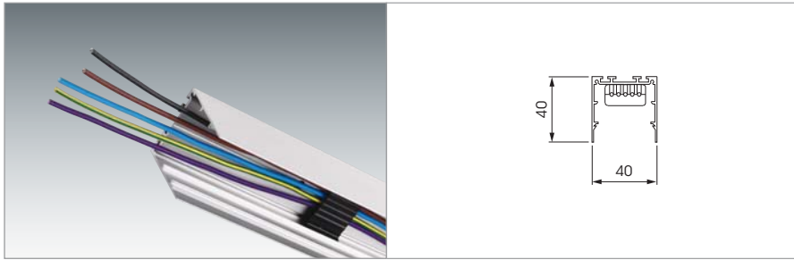
Aluminium-Profiltschiene 40x40mm, farblos eloxiert, mit Durchgangsverdrahtung 5x1,5mm 2 . Sonderlängen auf Anfrage.
