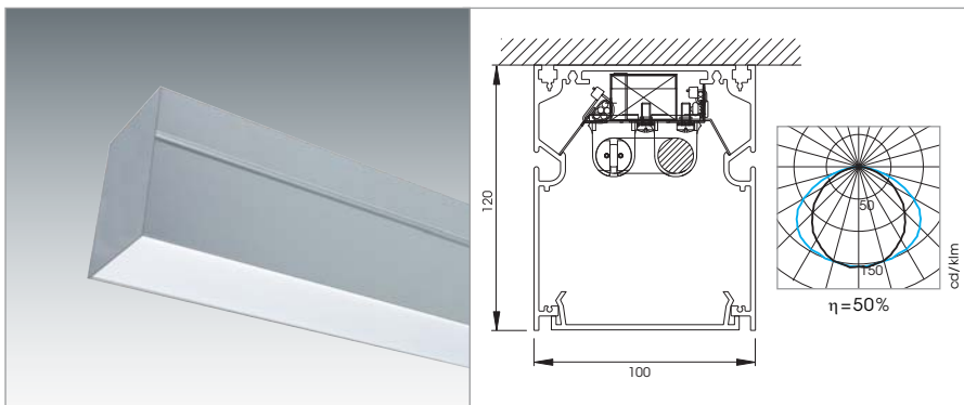
Alternativ: Leuchteneinsatz mit satiniertes Abdeckung für OM 76H zum Erzielen einer gleichmäßigen Ausleuchtung. [Art. No. siehe Seite 2.21]
