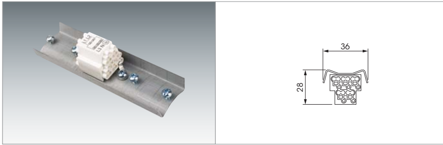
Profilverbinder mit Klemme 5x1,5mm 2 .
