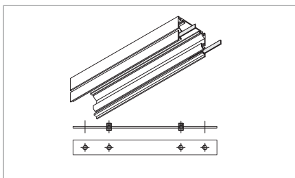
Längsverbinder.
