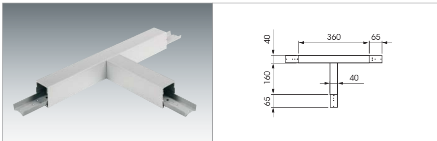
T-Verbinder, Aluminium-Profil farblos eloxiert.
