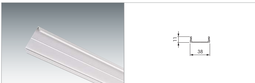
Blindabdeckung, Aluminium-Profiltschiene 40mm breit, farblos eloxiert, zum Einklippen in Profiltschiene 40x40mm. Sonderlängen auf Anfrage.
