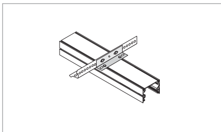
Abhänger zu Rostwinkel U 1040 bzw. Gewindestab.
