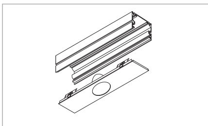
Downlight mit Abdeckung.
