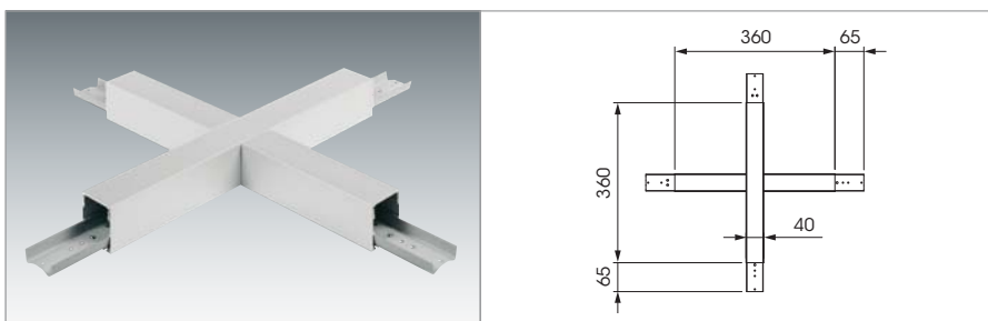
Kreuz-Verbinder, Aluminium-Profil farblos eloxiert.
