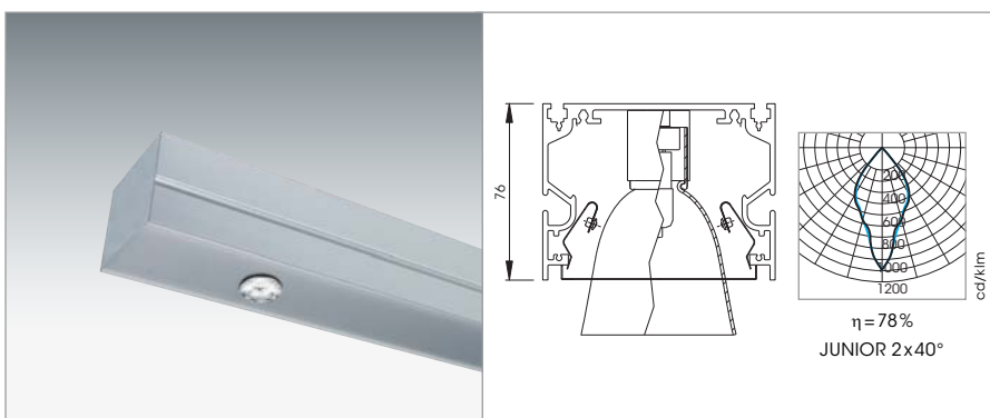
Downlight 20-35W / 12V mit elektronischem Vorschaltgerät. [Art. No. siehe Seite 2.21]
