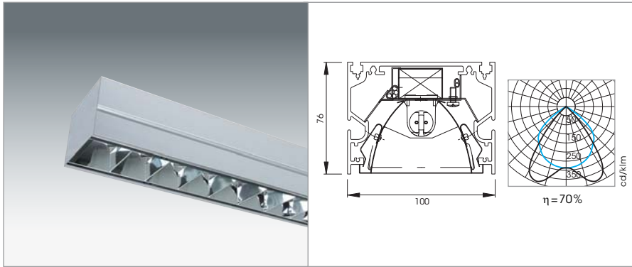
Leuchteneinsatz mit Parabolraster. [Art. No. siehe Seite 2.21]
