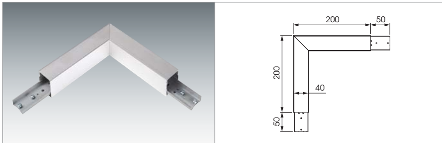
Eckverbinder, Aluminium-Profil farblos eloxiert.
