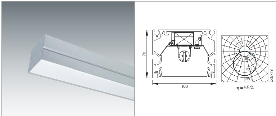
Leuchteneinsatz mit satiniertes Abdeckung. [Art. No. siehe Seite 2.21]
